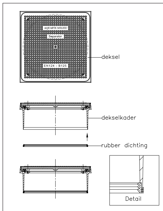
Afbeelding 4. Deksel en dichting
