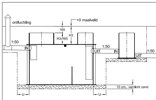
Afbeelding 3. Inbouw.
