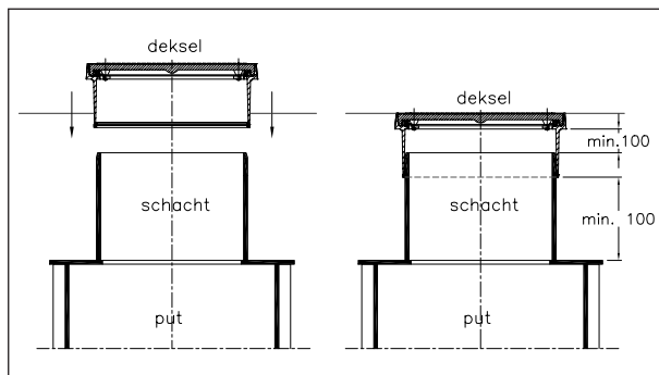
Afbeelding 5. Montage deksels
