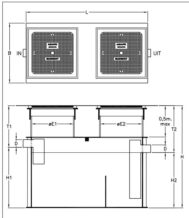
Afbeelding 2. Maattekening
